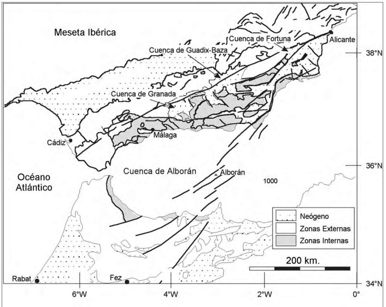
Figura 1. Situación de la cuenca de Fortuna en el contexto geotectónico de la cuenca de Alborán y arco de Gibraltar.
