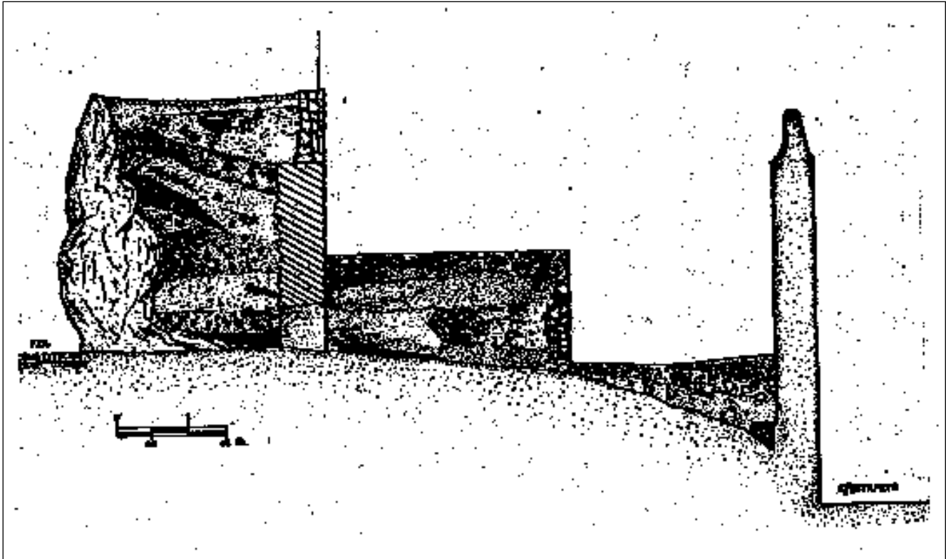
Fig. 7. Patio de Los Fajardo: Sección arqueológica a-b.
